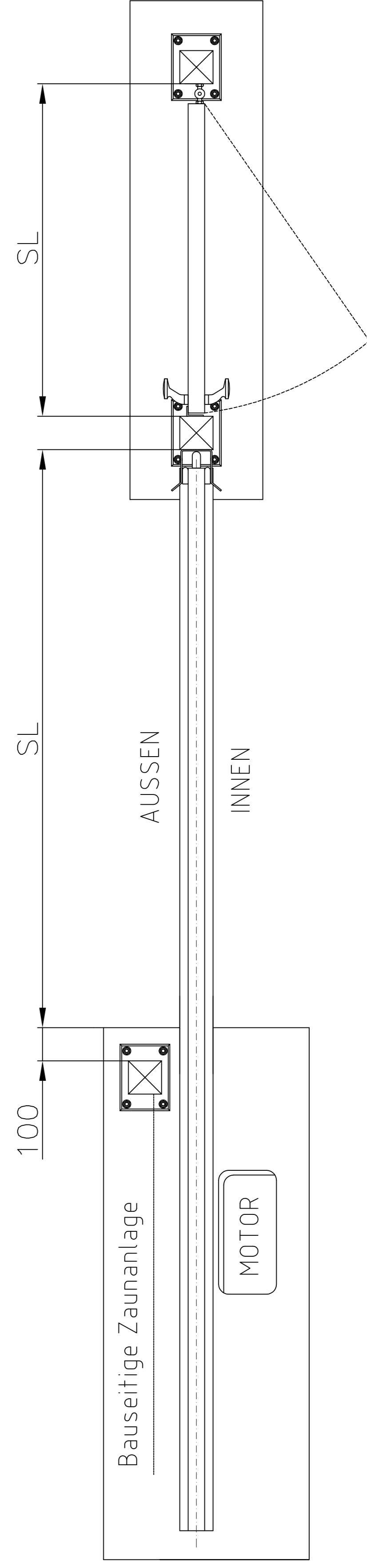
Einbausituation A1
