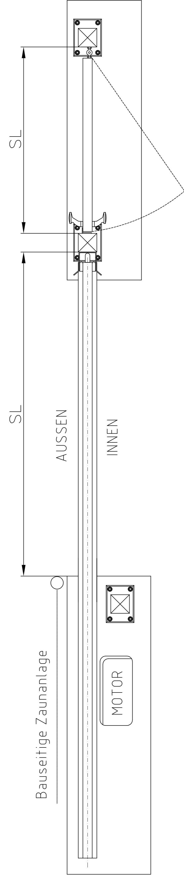
Einbausituation A2
